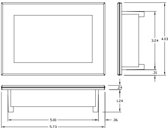
ST3™ Dimensions
